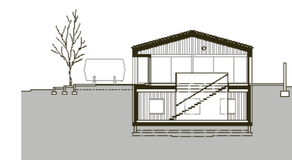
Querschnitt | Section
